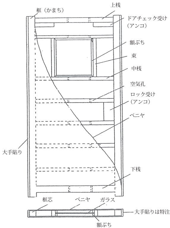
フラッシュドアの構造
